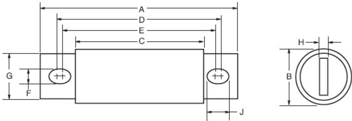
Fig. 1: 35-2000A
